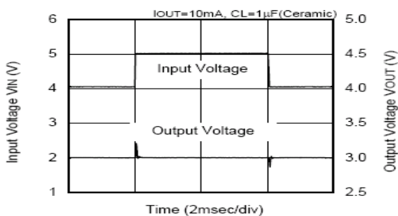
输入瞬态响应
